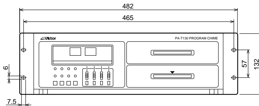
EIA用ラックマウント金具取付時(縮尺: 1/4)
